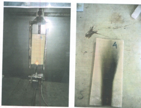
Thử nghiệm tính bất cháy Mẫu sau thử nghiệm bất cháy
